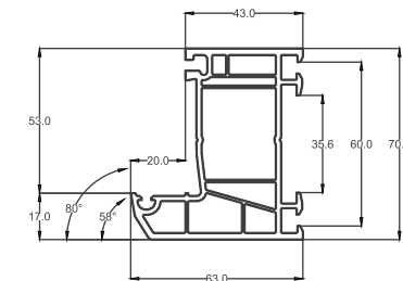
Профиль рамы арт. 7501
