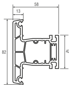
Профиль импоста арт. 5803
