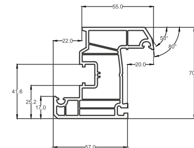
Профиль створки арт. 7502
