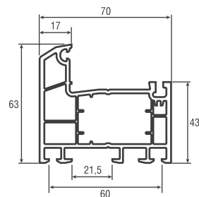
Профиль рамы арт. 7301
