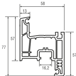
Профиль створки арт. 5802
