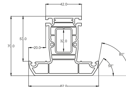
Профиль импоста арт. 7503
