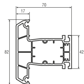
Профиль импоста арт. 7303
