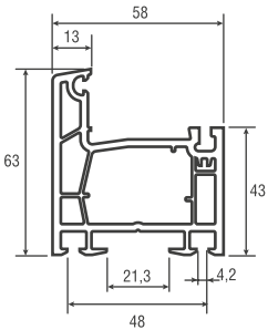
Профиль рамы арт. 5801
