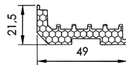
Термовставка фальца заполнения
