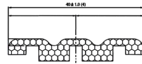
Термовставка фальца заполнения
